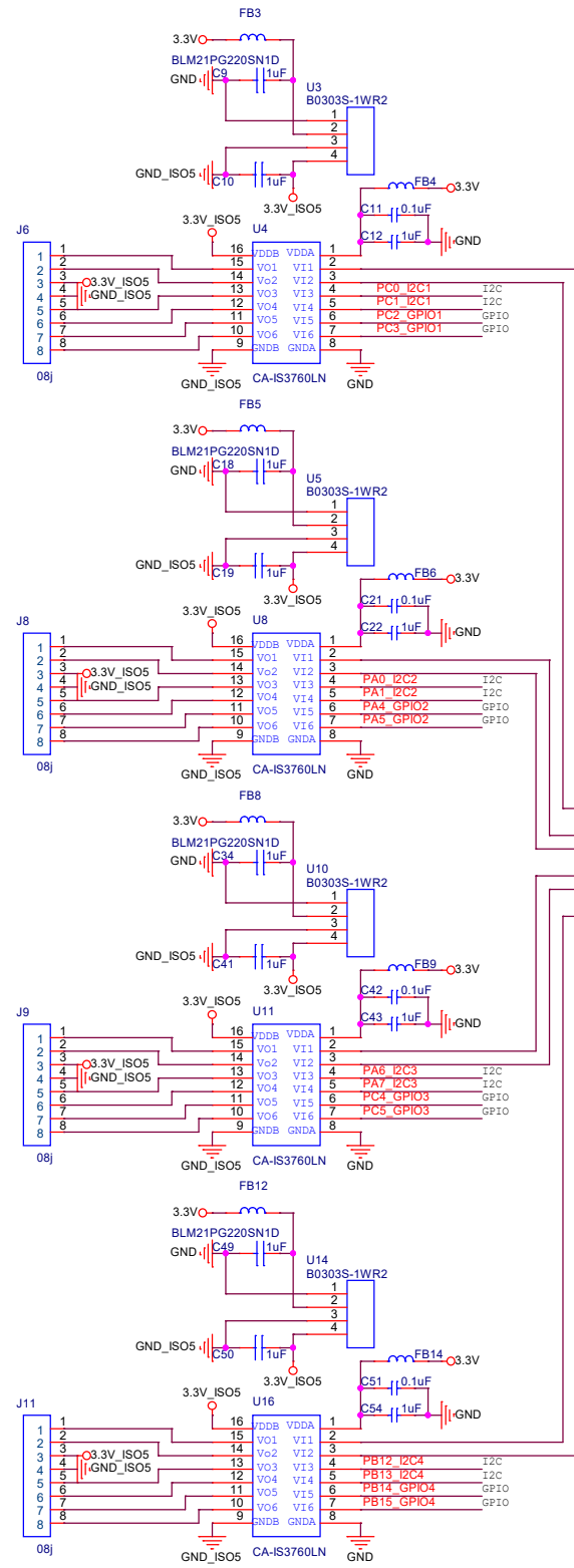
协议接口
