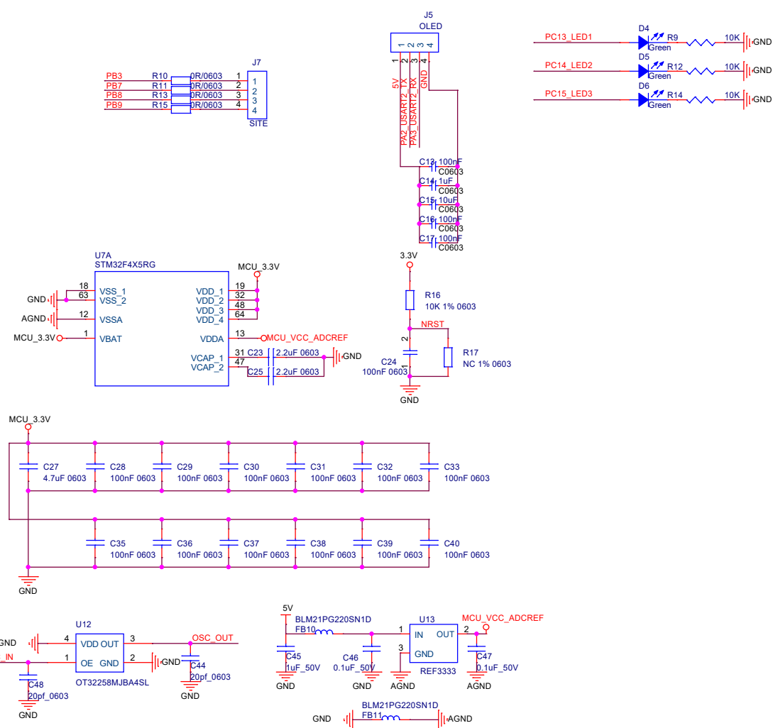
OLED屏
