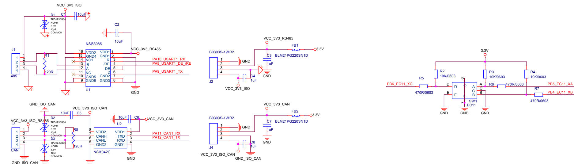
485和CAN通讯
